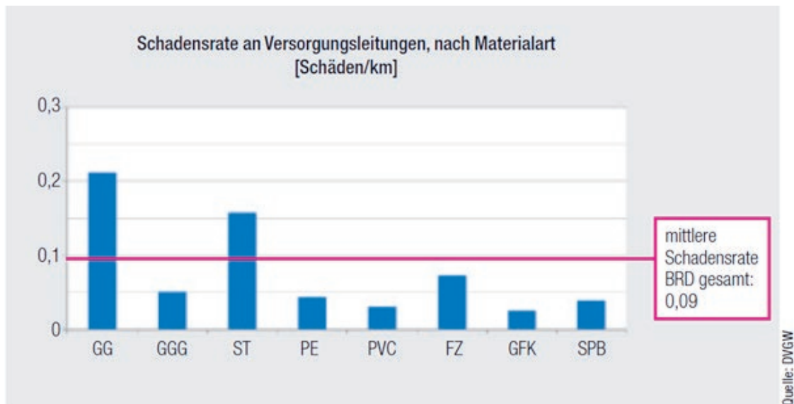
Wasserversorgung Deutschland (Versorgungsleitungen 2010-2012)
