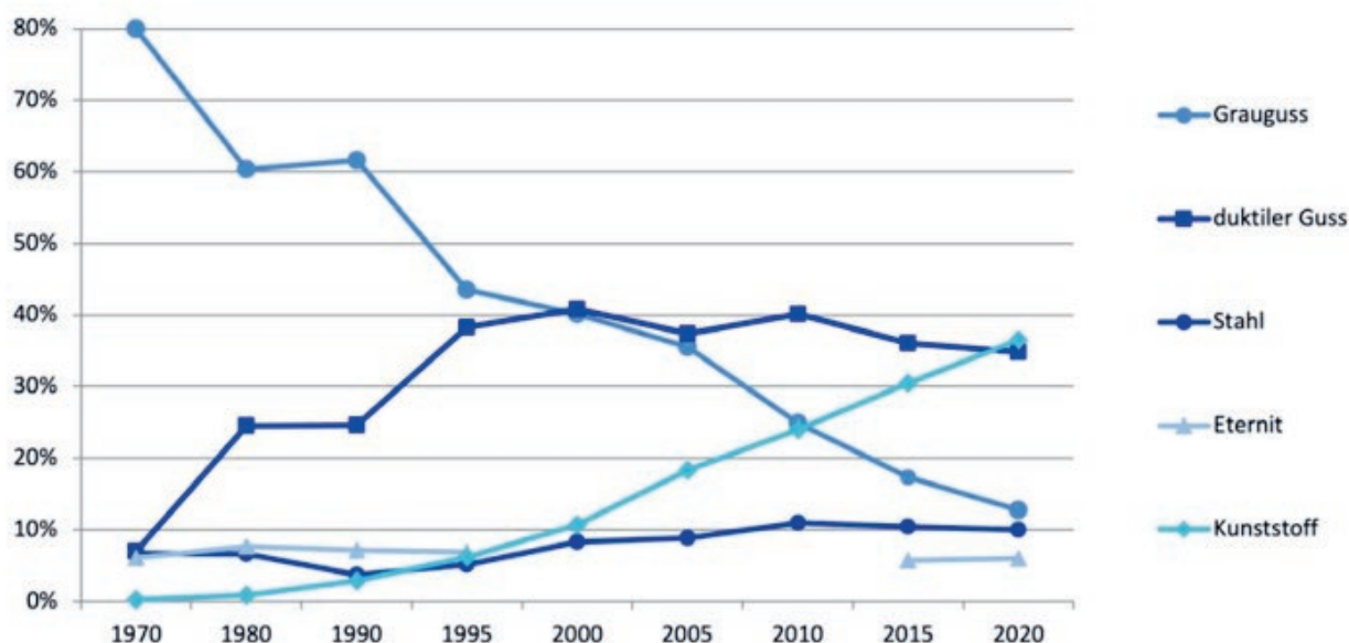
Abb 1.8 Rohrleitungsmaterialien seit 1970 (inkl. Hausanschlussleitungen) Fig. 1.8 Matériaux de conduites depuis 1970 (y compris conduites de raccordement)
